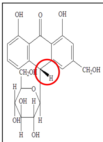
蘆薈苷 (Aloin)
